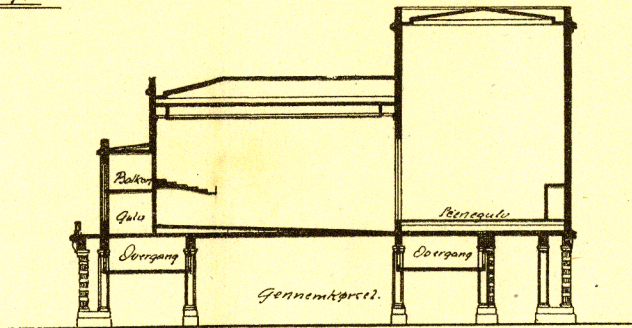
Tunnel. Længdesnit.
