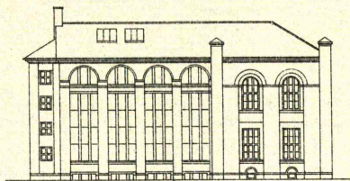
BIBLIOTEKSFLØJENS SYDSIDE
