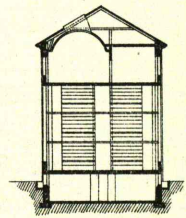
TVÆRSNIET GENNEM BIBLIOTEKSFLØJ.
